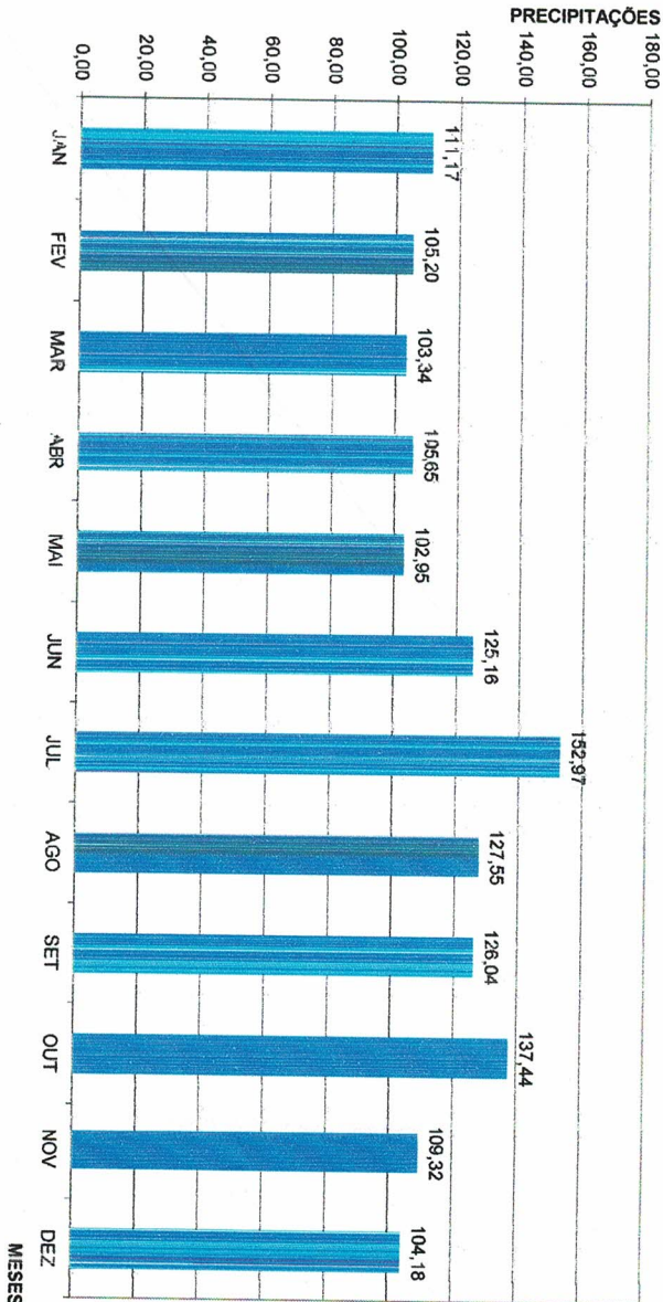
Figura 5 - Histograma da média histórica das precipitações totais mensais.
